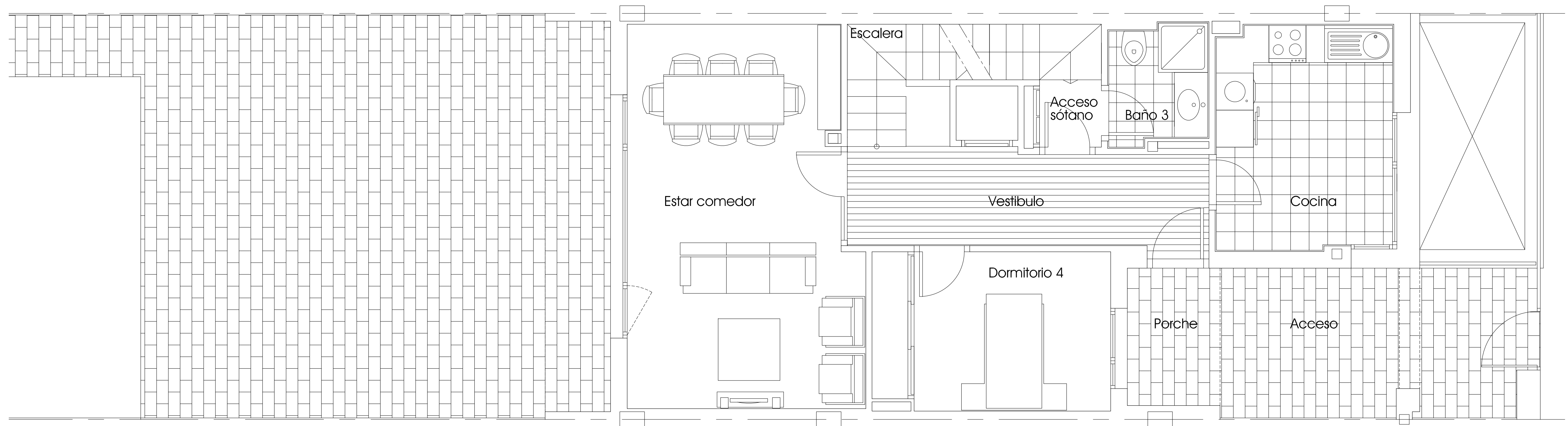
Planta Baja
