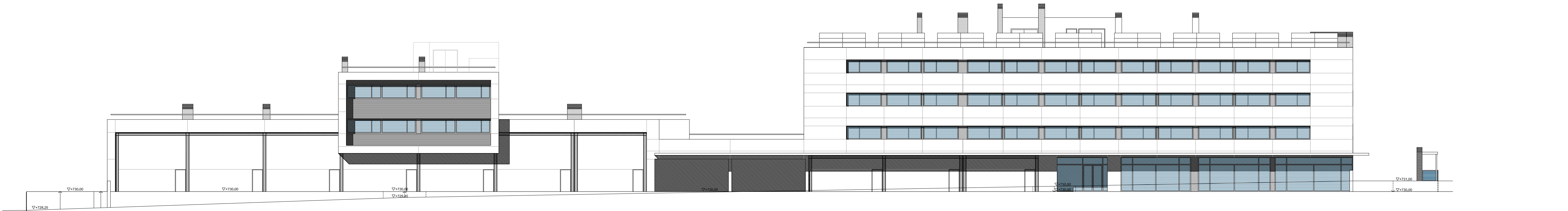
ALZADO SUR CALLE ORO
