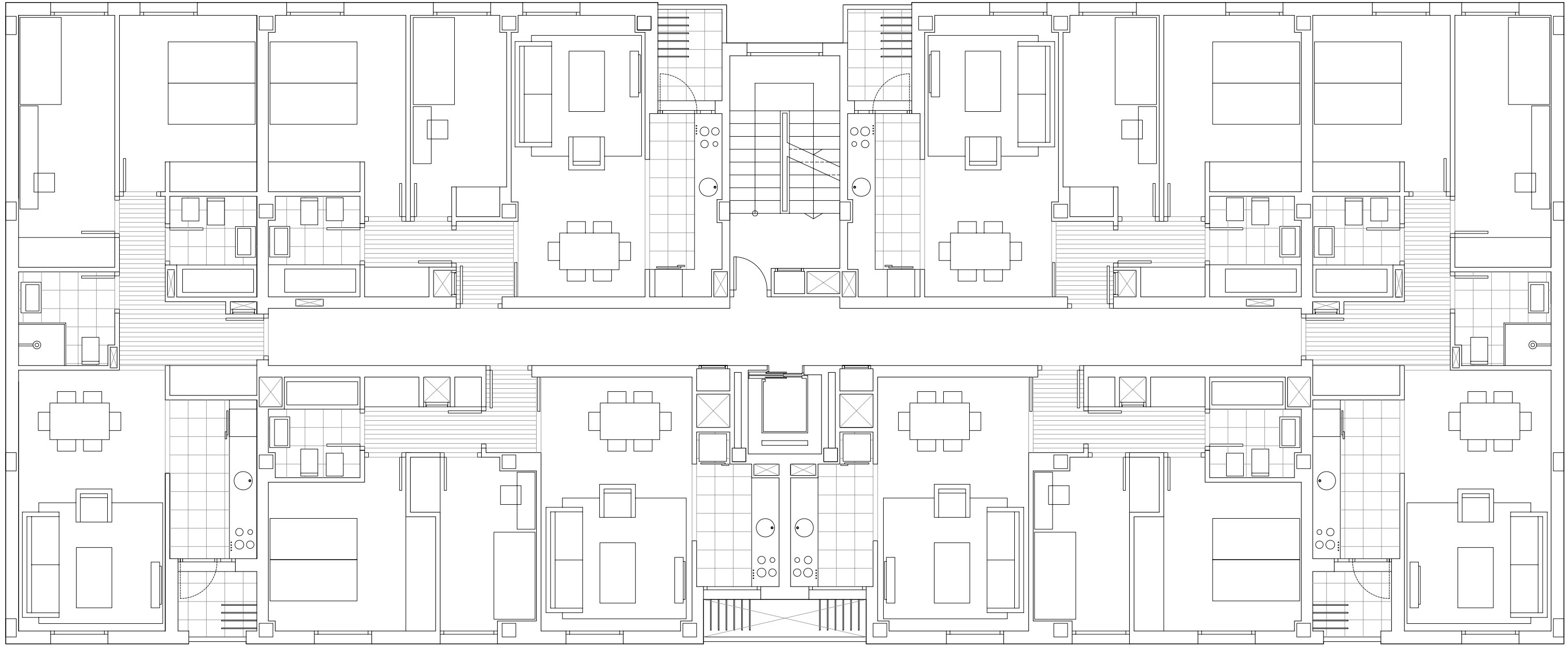
PLANTA TIPO
